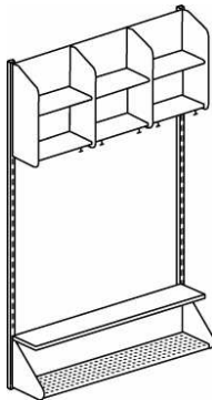
Kombi D -Kapphylla -Skohylla -Sittbänk -Väggskenor
